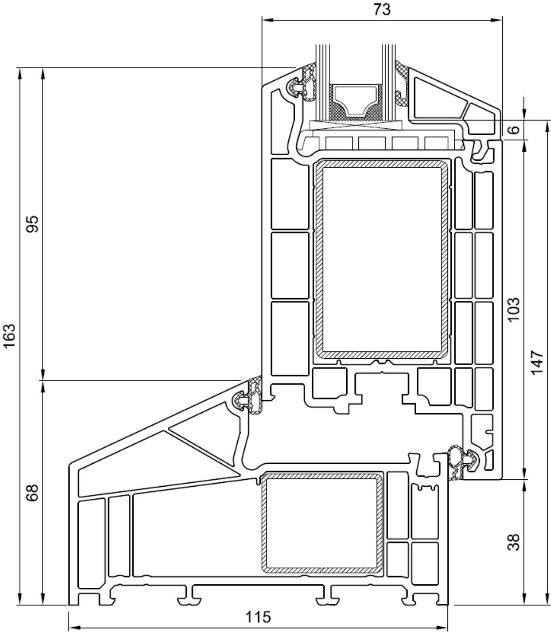
Kozijn zonder aanslag en deur binnen draaiend "verdiept profiel Creon"
